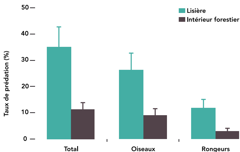
Figure 1 : Comparaison des taux de prédation moyens de ravageurs de cultures en lisière et à l'intérieur des massifs.
